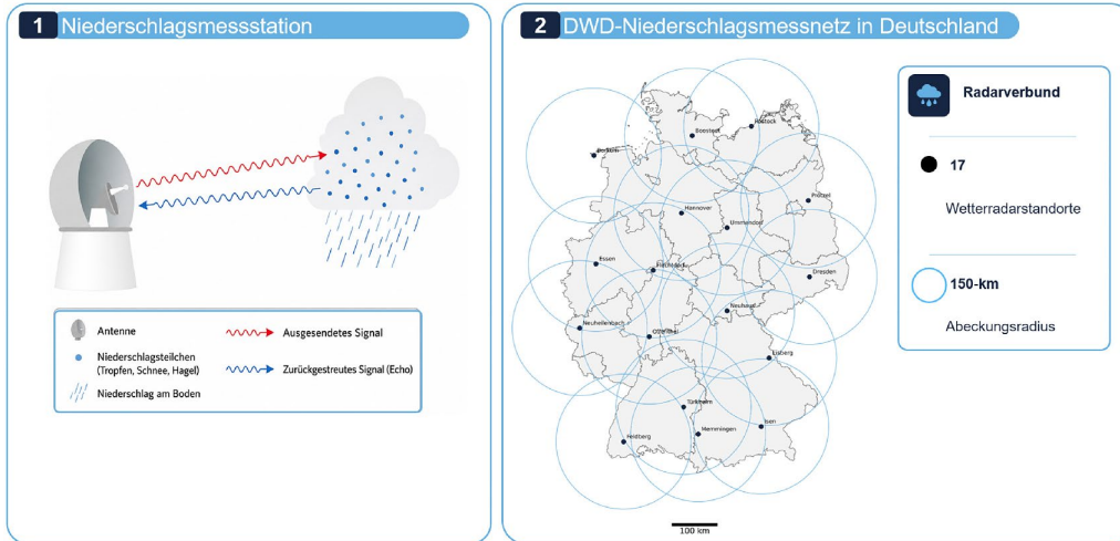
Abb. 03: Schematische Funktionsweise von Wetterradar und Radarverbund DWD [Quelle: Meteovise]
