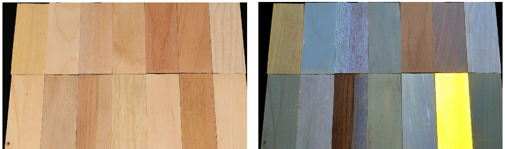
Abb. 01: Unterschiedliche Holzarten im Normalbild (links) und im UV-angeregten Fluoreszenzbild (rechts). Die starke Fluoreszenz von Robinie (unten, zweite Tafel v.r.) gilt als Alleinstellungsmerkmal, aber auch alle anderen Hölzer fluoreszieren. Nicht-fluoreszierende Gegenstände wären schwarz im Fluoreszenzbild. [Foto: Dr. F. B. Peters]
