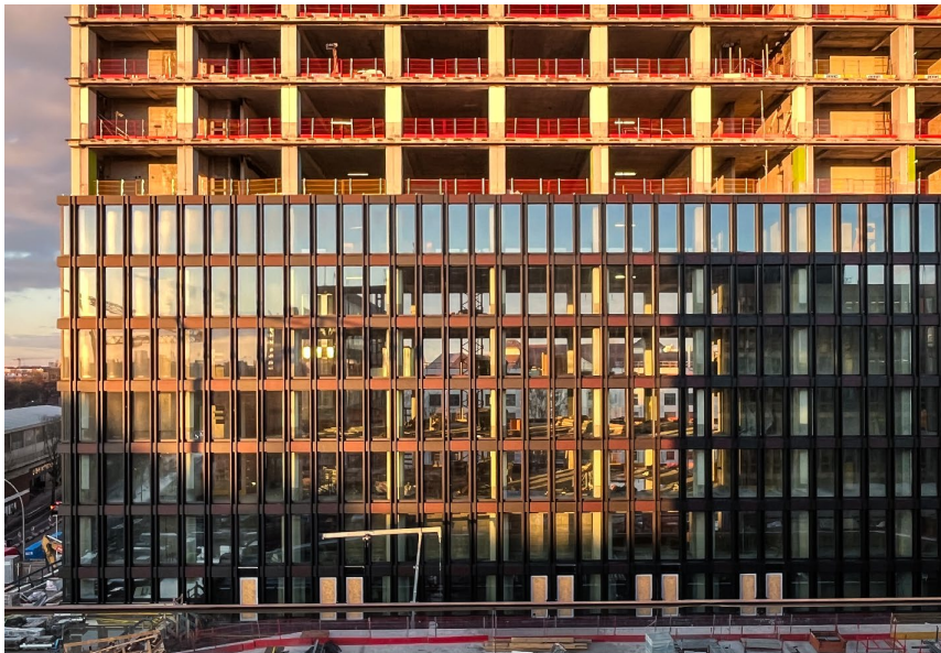
Abb. 04: Fassadenbaustelle [Foto: Konrad Hofmann]
